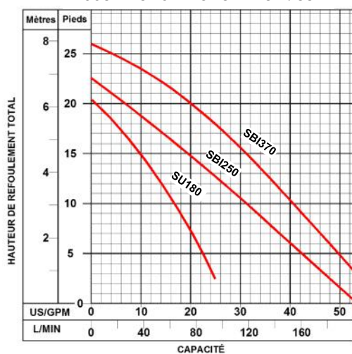
COURBES POMPAGE SÉRIE SBI / SU
