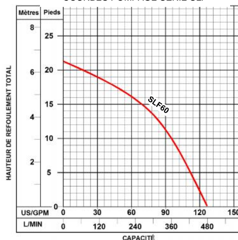
COURBES POMPAGE SÉRIE SLF
