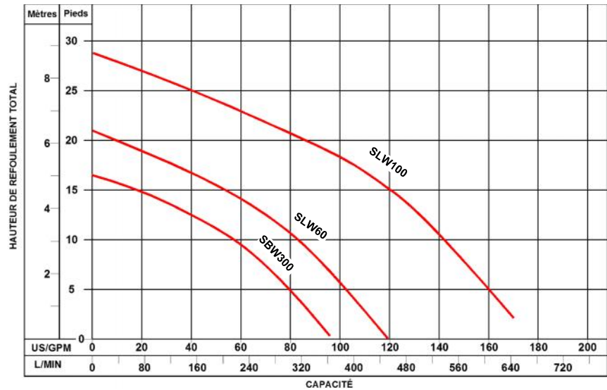
COURBES POMPAGE SÉRIE SBW / SLW
